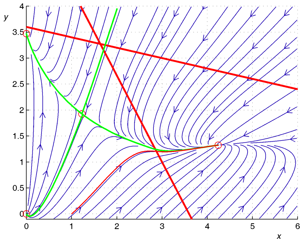
Рис. 3. Благоприятный вариант развития
