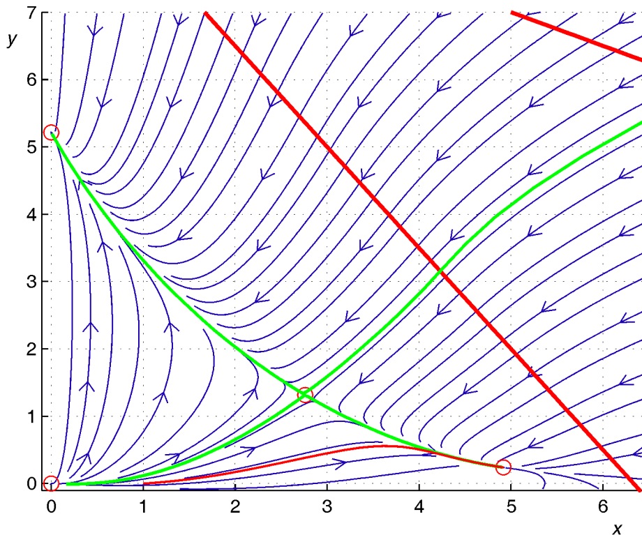
Рис. 2. Благоприятный вариант развития
