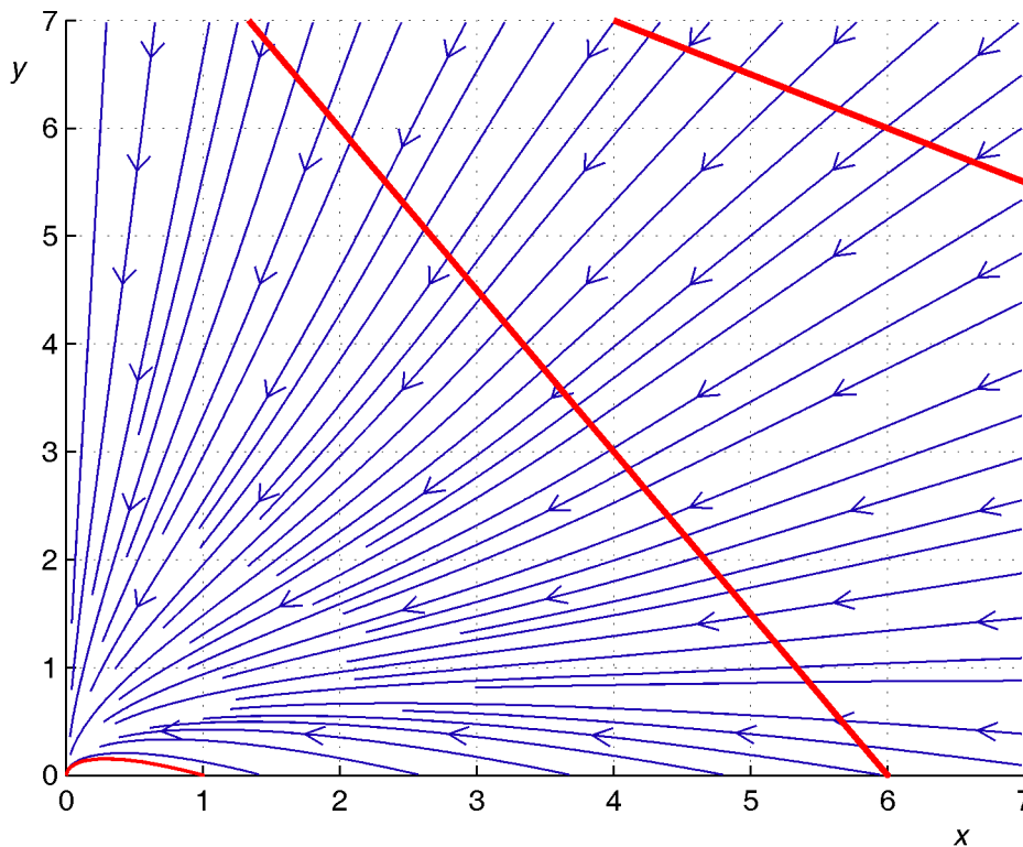
Рис. 6. Неблагоприятный сценарий — полное вымирание популяционной системы
