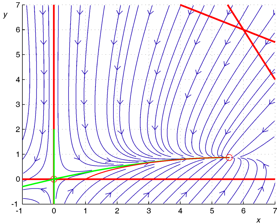
Рис. 5. Благоприятный сценарий — преобладание нормальных клеток
