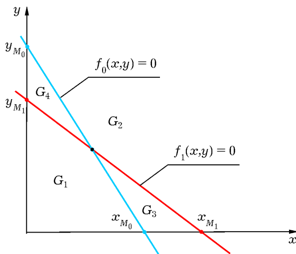
Рис. 1. Вариант разбиения множества G
