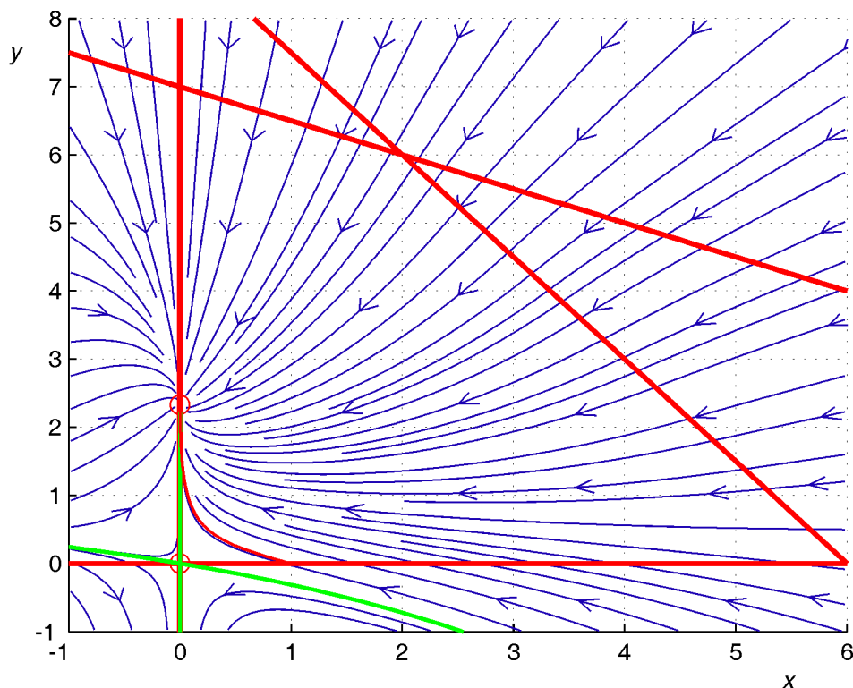
Рис. 4. Неблагоприятный сценарий — вымирание популяций нормальных клеток
